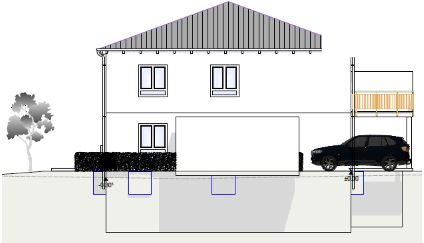
Ansicht Nord-Westen
